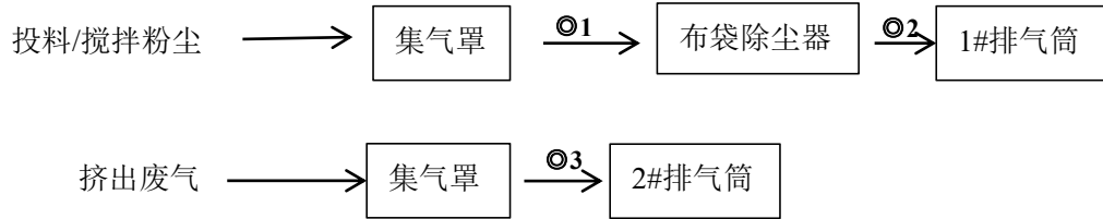
图 3-2 废气处理工艺流程图
