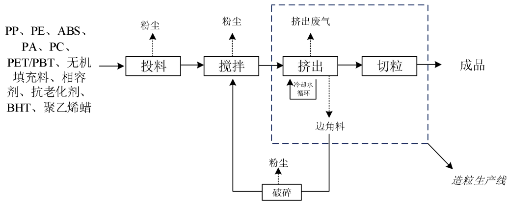
图 2-3 生产工艺与产污情况
